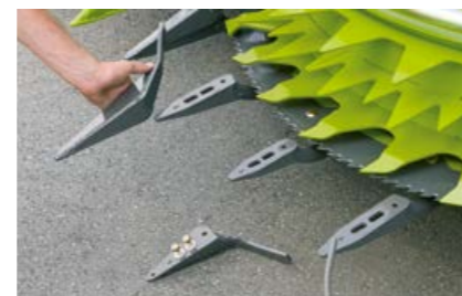
Demontierbare Einweiserfinger verbessern das Aufheben von Lagermais.
